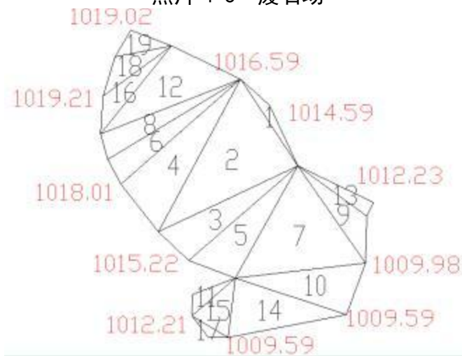
图 4-1 三角网法计算废石量
